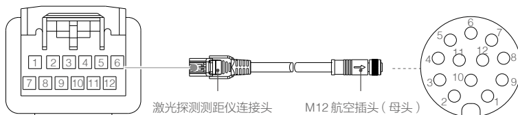
图 2.1.1 航插电源网口线
