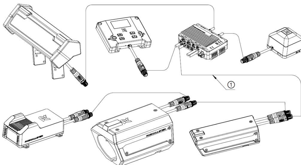
图 3-7 电源管理模块接口示意图
