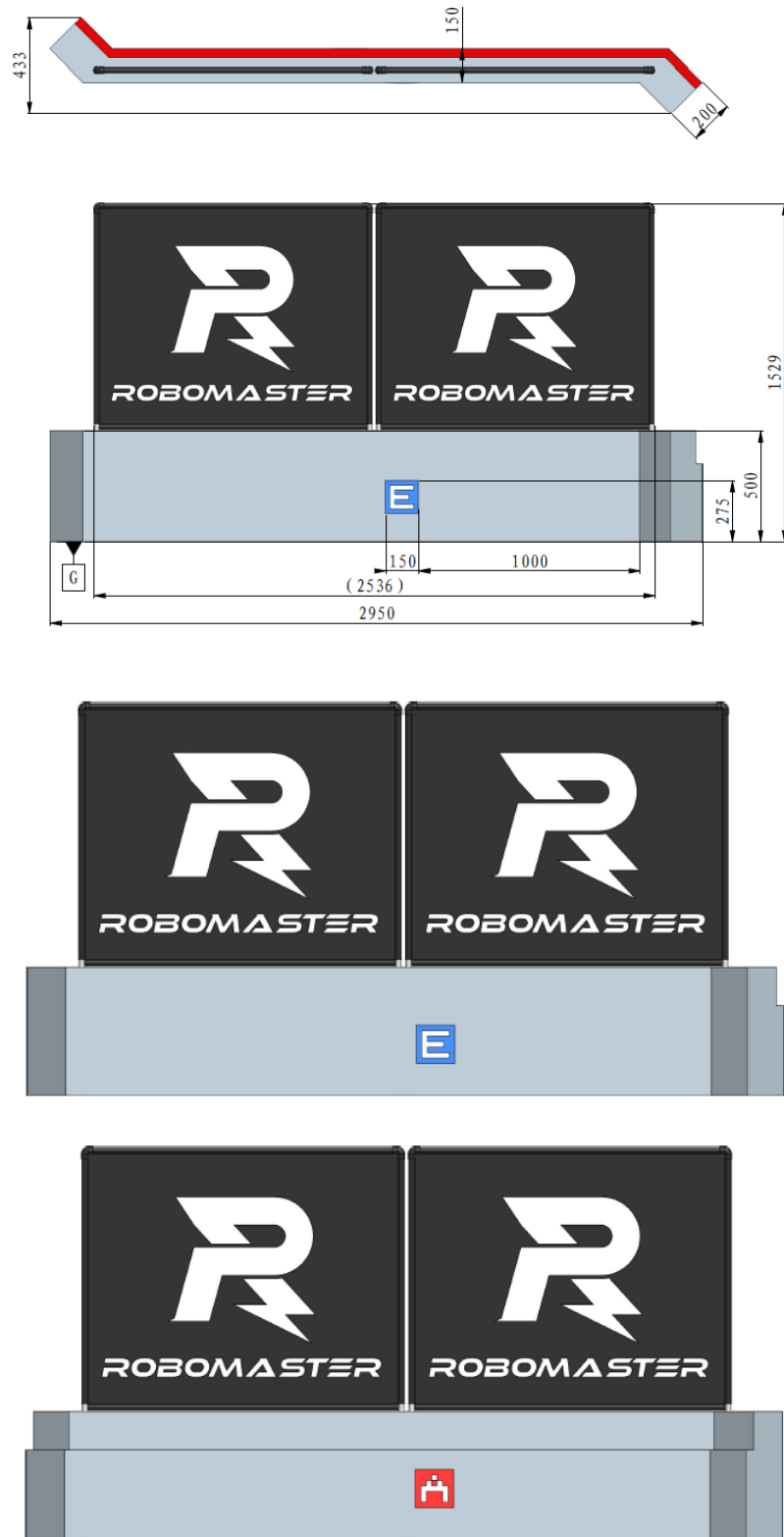
图 5-11 木质场地掩体示意图
