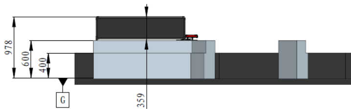
图 5-8 木质场地启动区示意图
