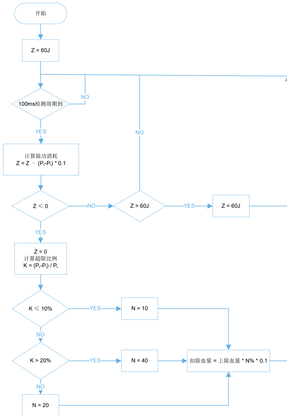
图 4-4 步兵机器人和英雄机器人底盘功率检测及扣血逻辑图
