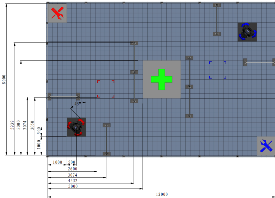
图 5-3 3V3 对抗赛拼接场地尺寸示意图
