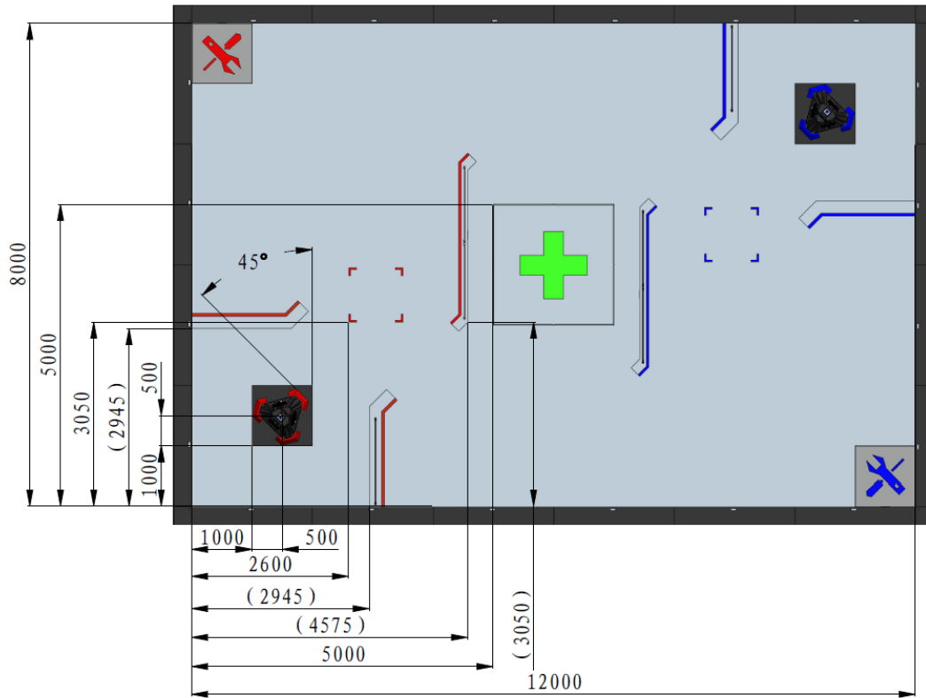
图 5-6 3V3 对抗赛木质场地尺寸示意图
