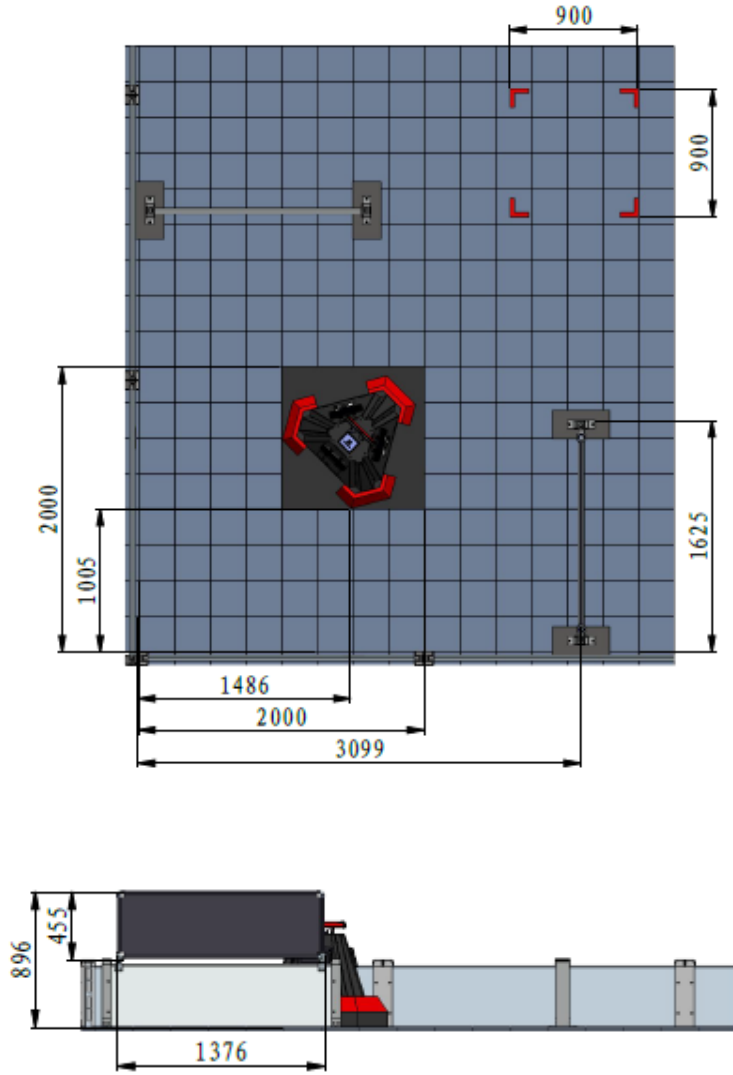
图 5-7 拼接场地启动区示意图
