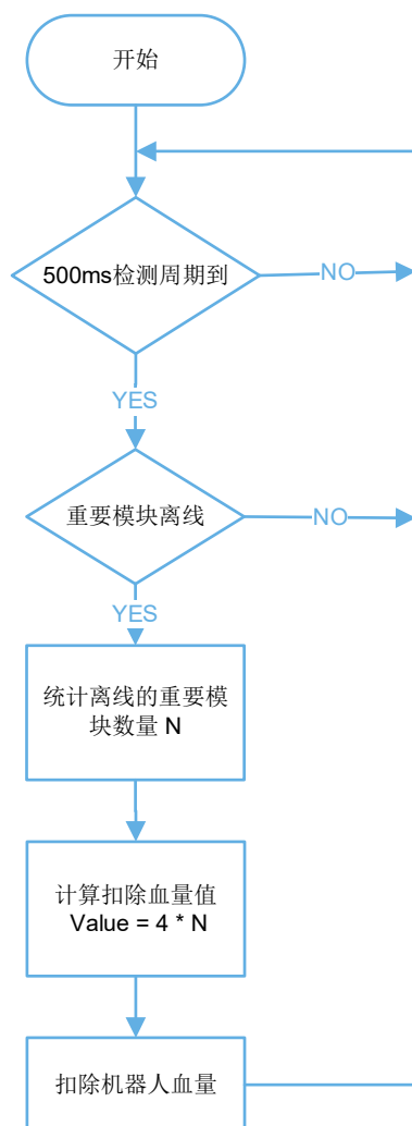
图 4-6 裁判系统重要模块离线扣血机制
