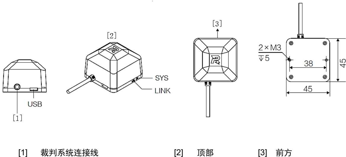
图 3-43 定位模块示意图
