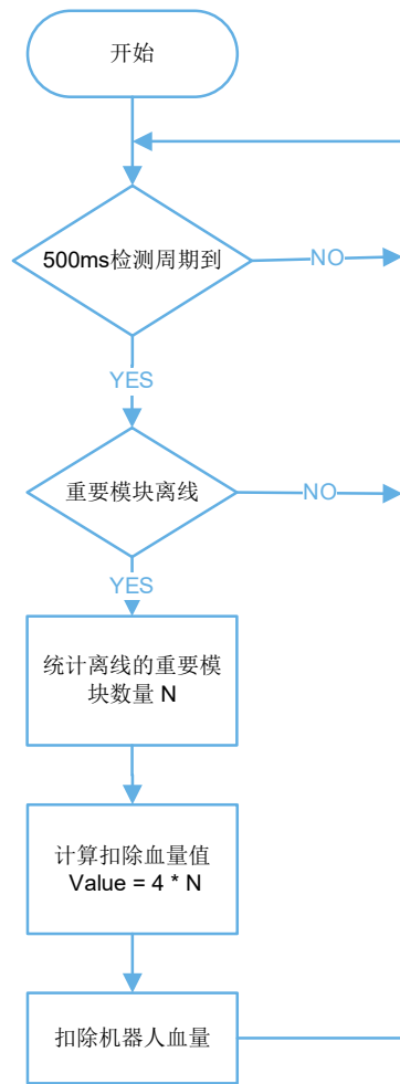
图 4-4 裁判系统重要模块离线扣血机制
