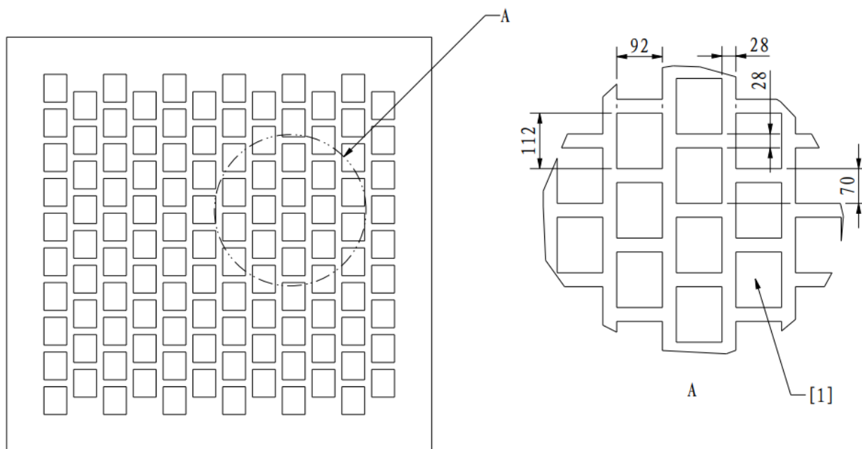
图 5-9 中心增益点示意图
