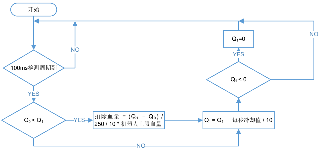
图 4-2 枪口热量冷却逻辑图
