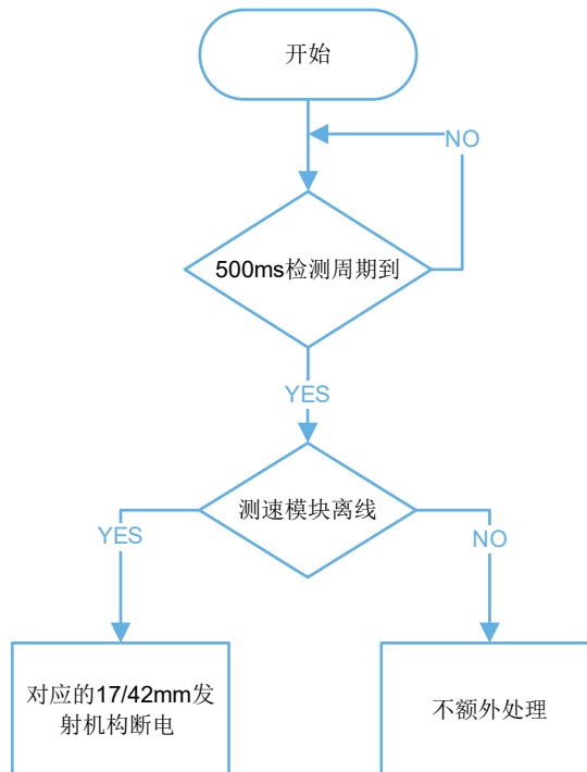
图 4-5 测速模块离线断电机制
