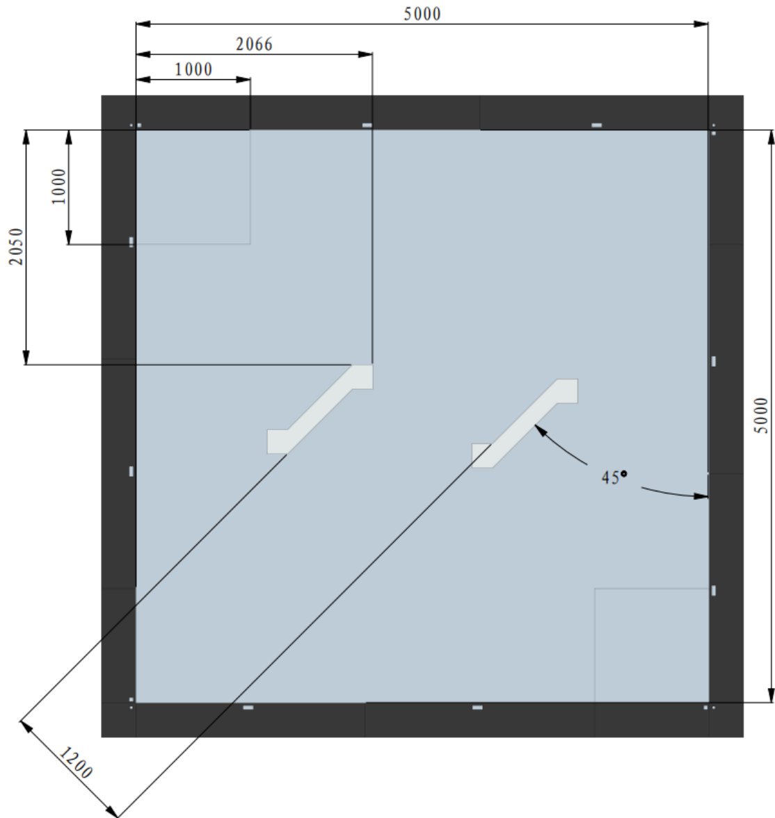
图 5-16 步兵对抗赛木质场地尺寸示意图
