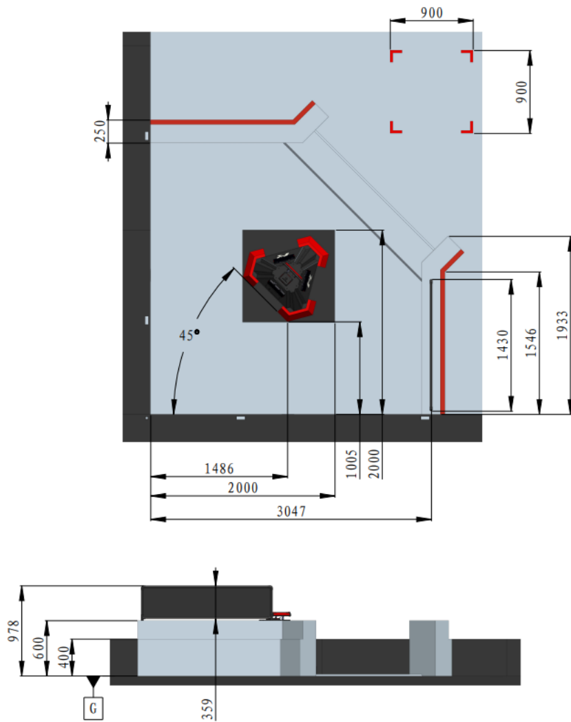
图 5-4 木质场地启动区示意图
