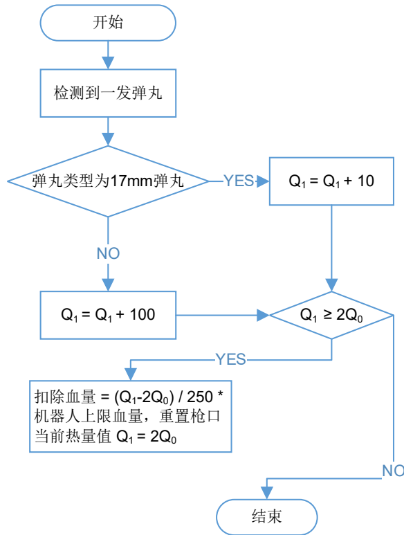
图 4-1 枪口热量超限计算逻辑图
