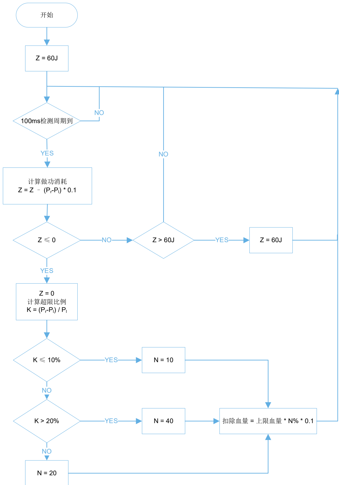
图 4-3 英雄、步兵、哨兵机器人底盘功率检测及扣血逻辑图
